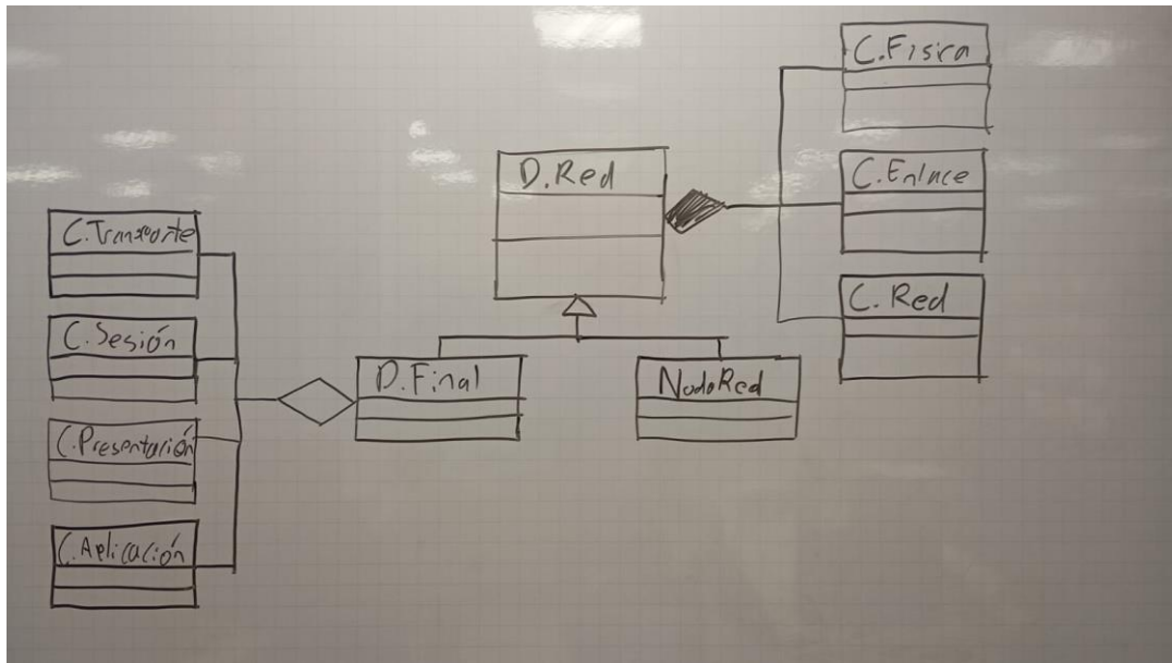
Ilustración 4 Diagrama de clases de potencial estructura de los elementos de red
